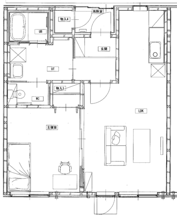
1LDK間取り図 52.79㎡ (参考)
